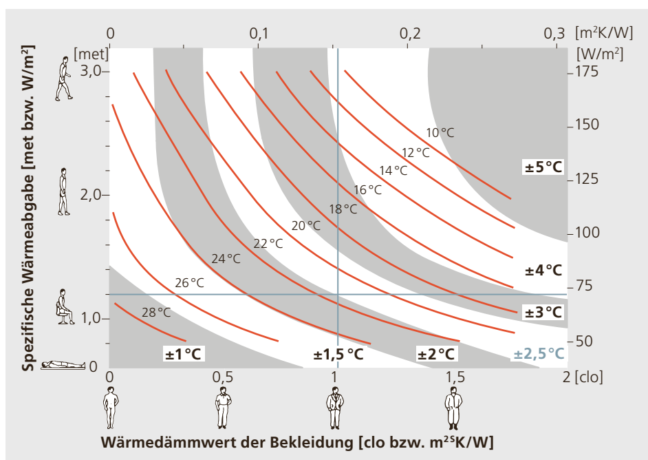
Abbildung 2.3: Optimale Raumtemperatur in Abhängigkeit von Kleidung und Aktivität nach ISO 7730.
