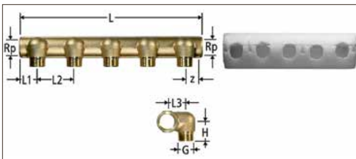
Abbildung 3.16: Auch Wohnungsverteiler für Warmwasser sollen gedämmt sein. (Quelle: R. Nussbaum AG)
