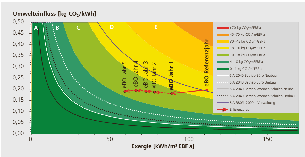
Abbildung 4.6: NSE-Diagramm mit Grenz- und Zielwerten aus den SIA-Normen. Primärenergiefaktoren und Treibhausgasemissionswerte für Heizöl EL sowie den Schweizer Strommix nach KBOB.
