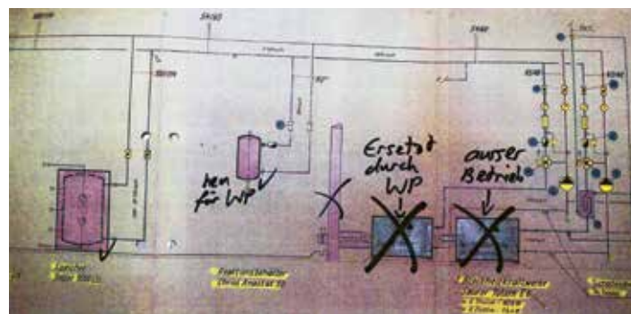
Abbildung 6.4: Ausschnitt aus dem Original-Prinzipschema der Heizungsanlage; wie zu sehen ist, wurde sie im Lauf der Zeit mehrfach angepasst. (Foto: Böhler, MTU GmbH)
