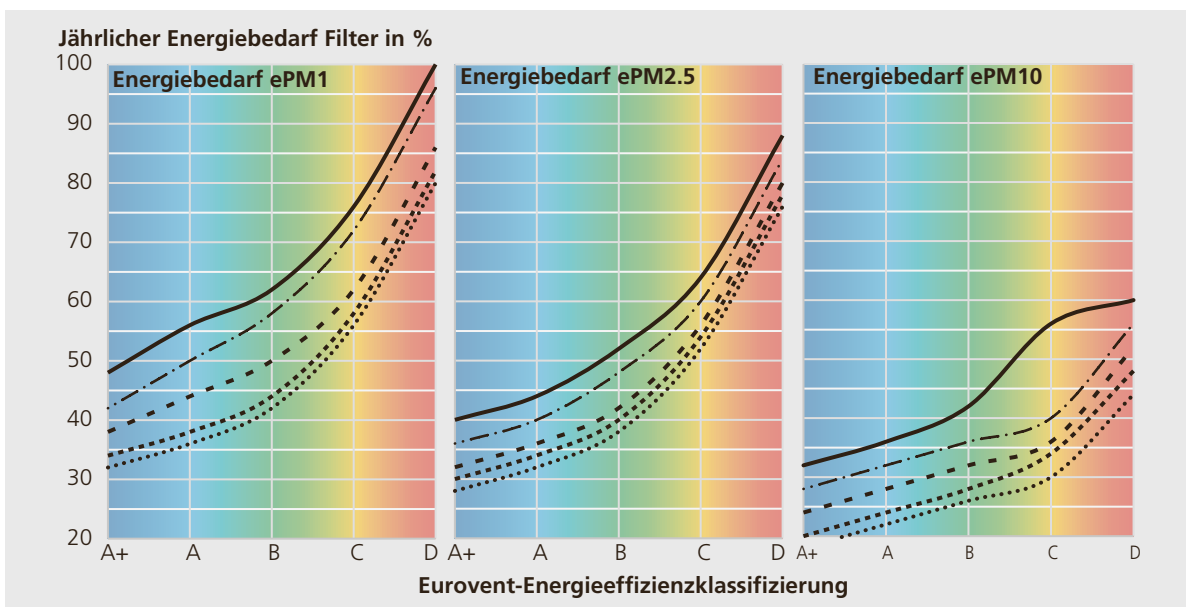
Abbildung 3.32: Vergleich des Jahresenergiebedarfs von verschiedenen Filtern in % (100% = höchster Bedarf) bei Standardprüf- und Berechnungsbedingungen nach Eurovent-Energieeffizienzklassifizierungen.
