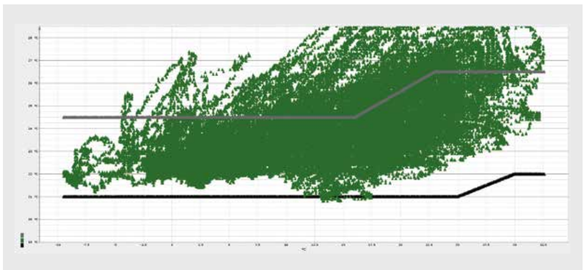
Abbildung 4.27: Raumlufttemperatur im Vergleich zu den Grenzwerten von SIA 180 (Raumlufttemperatur in Abhängigkeit der Aussenlufttemperatur). (Quelle: Enastra AG)
