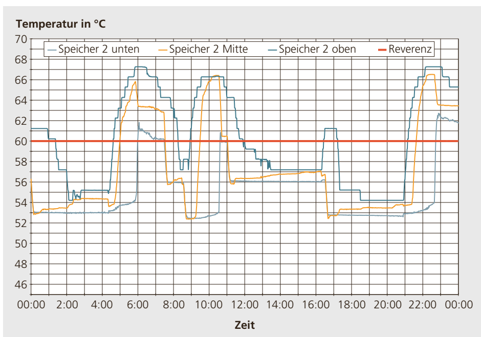
Abbildung 3.18: Temperaturverlauf im Warmwasserspeicher 2 (SP 2); rote Linie = Solltemperatur. (Quelle: S. Murchini, Büro für Messtechnik)
