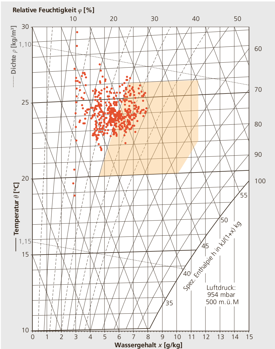
Abbildung 3.22: Beispiel Verwaltung – Darstellung Stundenwerte Raumtemperatur und Raumfeuchtemessung im h,x -Diagramm mit Behaglichkeitsbereich (hellorange).
