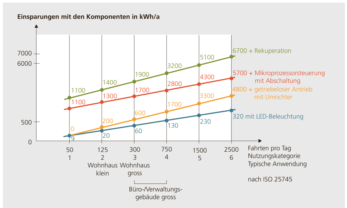
Abbildung 3.5: Kumulative Einsparungen pro Jahr aus verschiedenen Optimierungsmassnahmen an Aufzügen. (Quelle: Marcel Ackermann)
