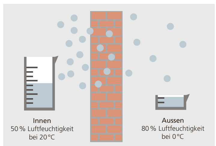
Abbildung 2.6: Der Partialdruck-Unterschied des Wasserdampfes zwischen Innen und Aussen ist der Treiber für die Dampfdiffusion in die Wand.
