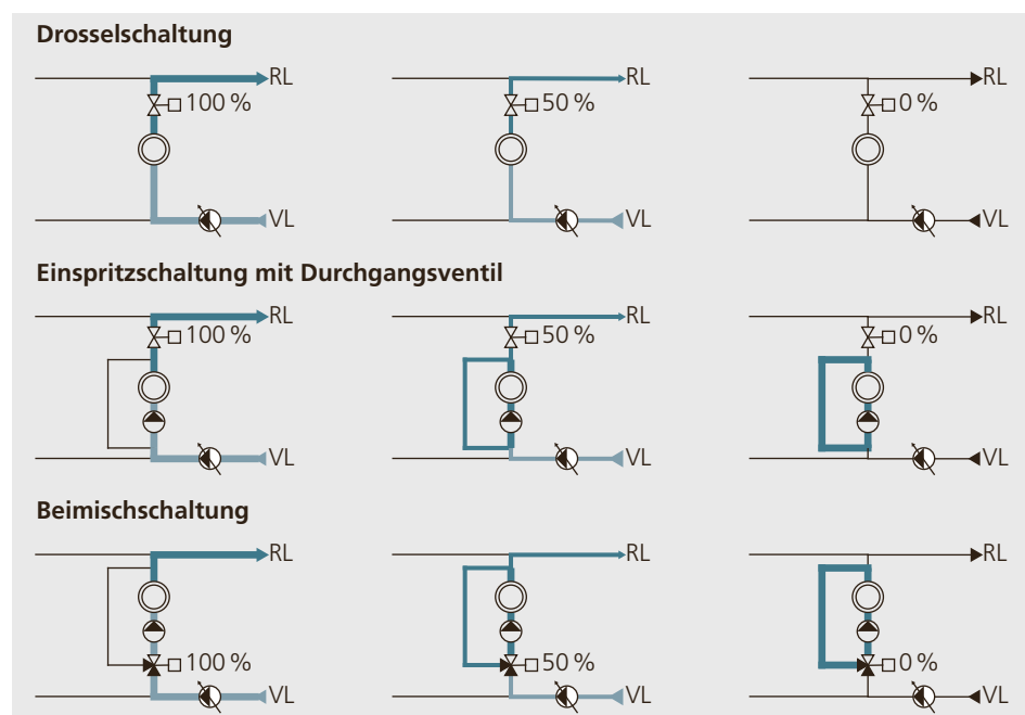
Abbildung 3.39: Mögliche hydraulische Schaltungen für Kälteverbraucher mit Teillastverhalten.
