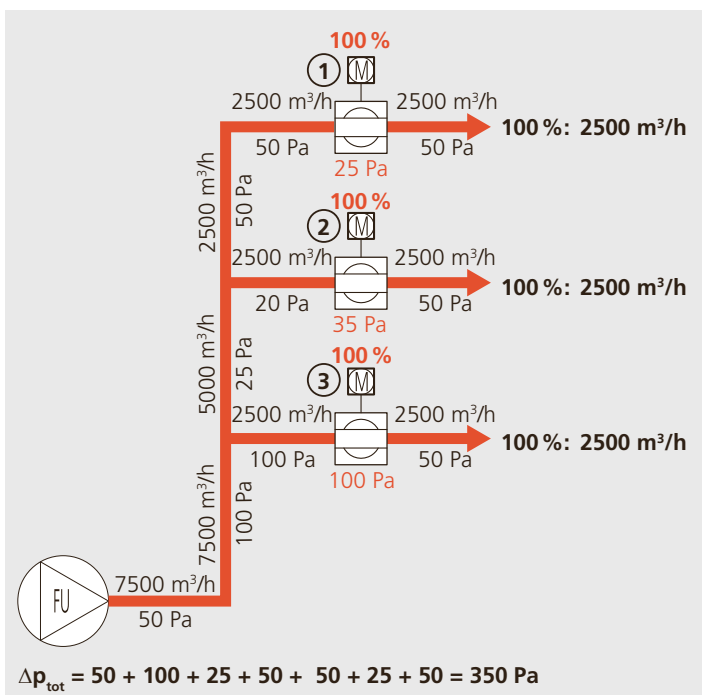
Abbildung 3.25: Beispiel Druck- erhöhung Ventilator, Auslegung 100%.
