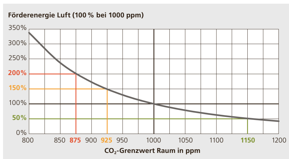
Abbildung 3.21: Theoretisches Verhältnis zwischen CO 2 -Konzentration in der Raumluff und Energiebedarf für die Luftförderung.
