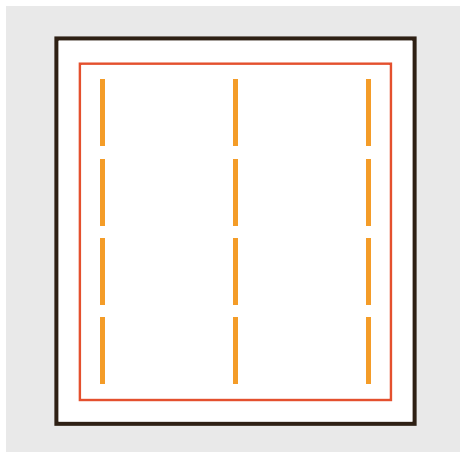
Abbildung 3.2: Grundriss des Schulzimmers (8 x 8,6 m), Anordnung der 12 Leuchten.
