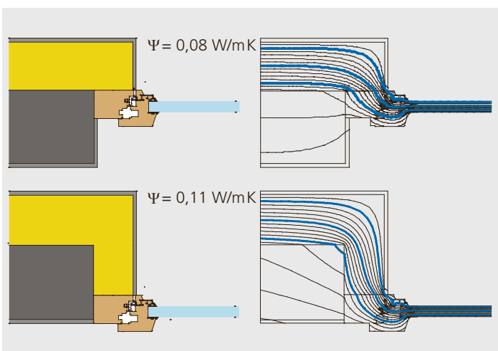
Abbildung 2.5: Beispiel für einen Fenstereinbau mit minimierter Wärmebrücke. (Quelle: EnFK)
