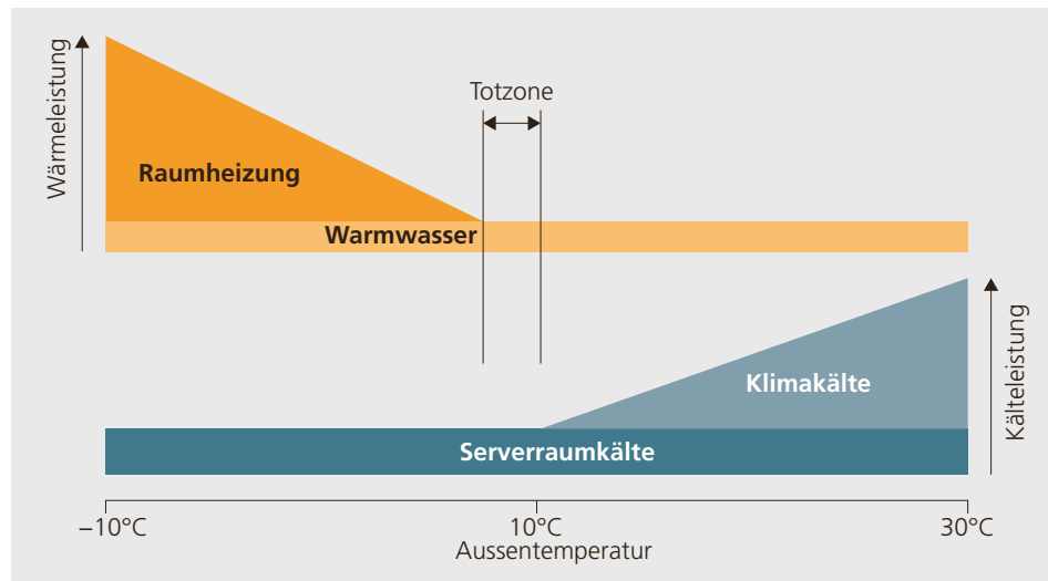
Abbildung 3.51: Echter Bedarf für Heizen und Kühlen, getrennt durch eine Totzone. (Quelle: Angelo Lozza, Lozza Energie und Gebäudetechnik)
