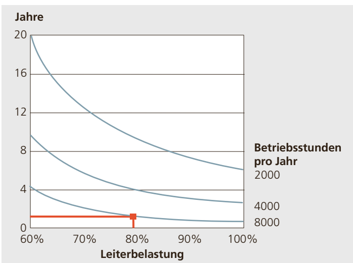
Abbildung 3.47: Amortisationsdauer von elektrischen Versorgungsleitungen in Abhängigkeit der jährlichen Betriebsstunden und der Auslastung in Prozent zur maximalen Normlast. (Quelle: Peter Bryner, Electrosuisse)
