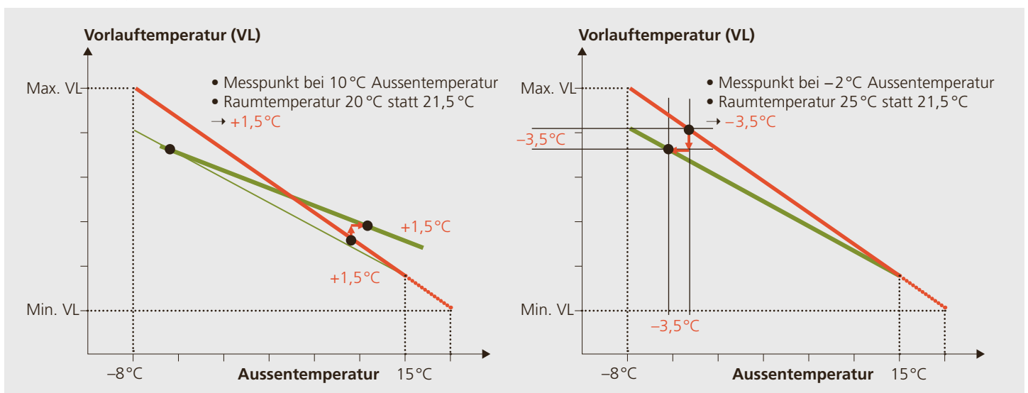
Abbildung 3.6: Vorgehen für Korrektur Heizkurve; rot: alte Heizkurve, grün: neue Einstellungen.
