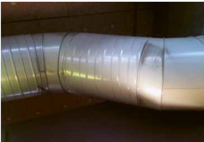
Abbildung 3.24: Leckagen bei Rohrverbindungen, hier anhand von Staubablagerungen sichtbar.
