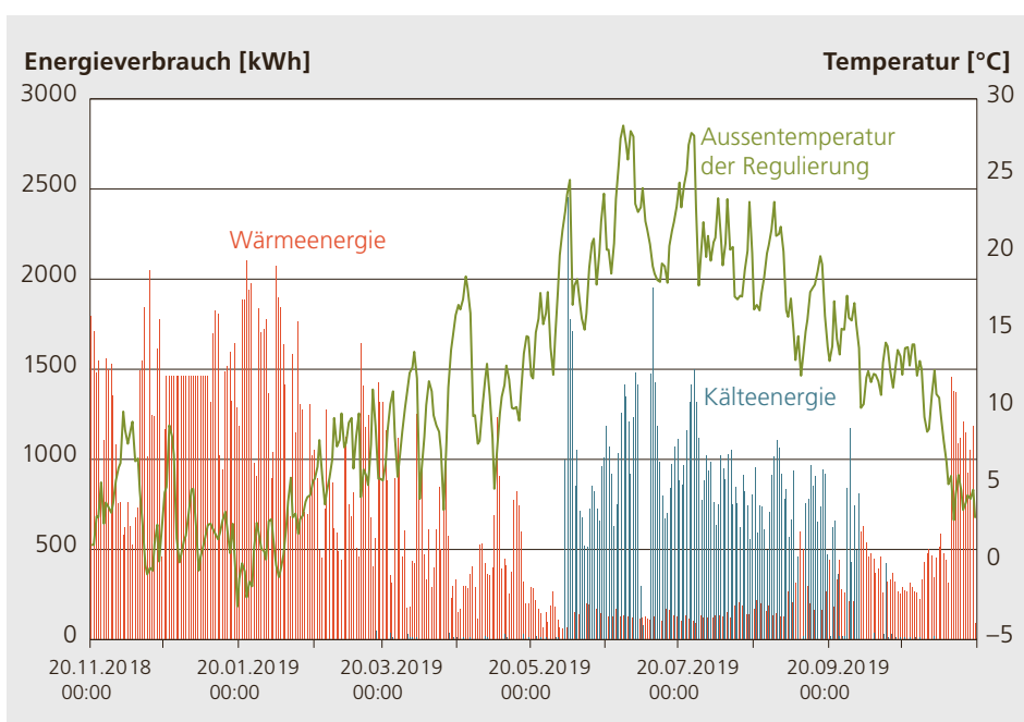
Abbildung 4.29: Übersicht über den jährlichen Wärme- und Kälteenergiebedarf mit Aussentemperaturverlauf. (Quelle: Enastra AG)
