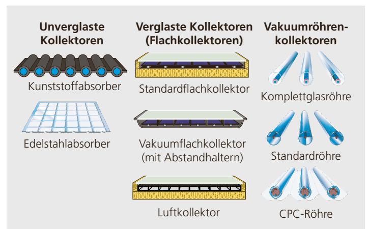
Abbildung 3.58: Bauarten Solar Kollektor. (Quelle: Dimensionierungshilfe Haustechnik, EnergieSchweiz)
