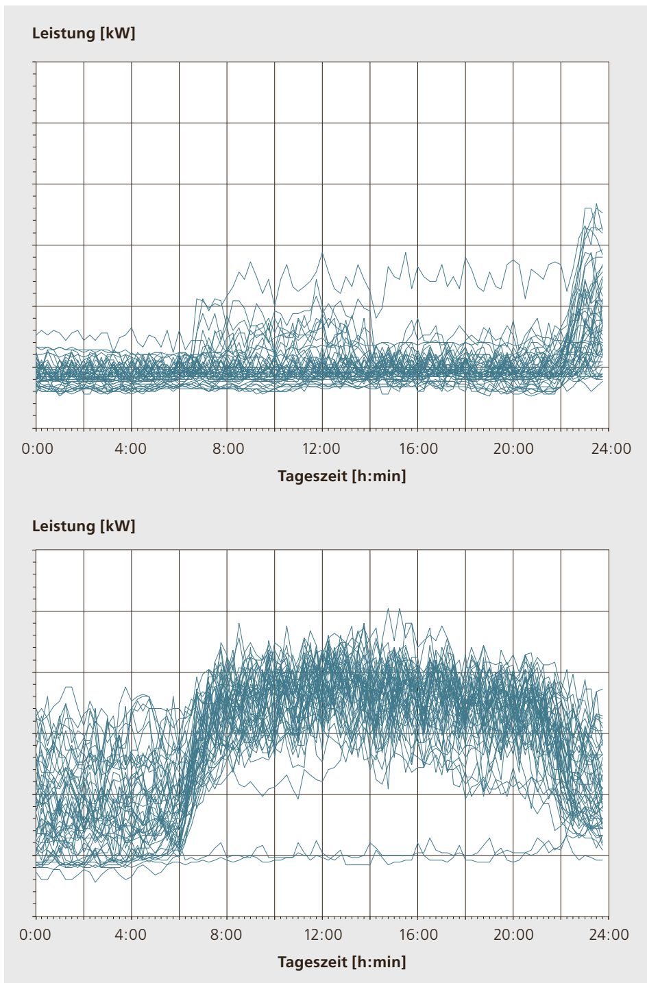
Abbildung 4.1: Überlagerte Tagesprofile des Stromverbrauchs eines Betriebs. Oben: sonntags, unten: montags.
