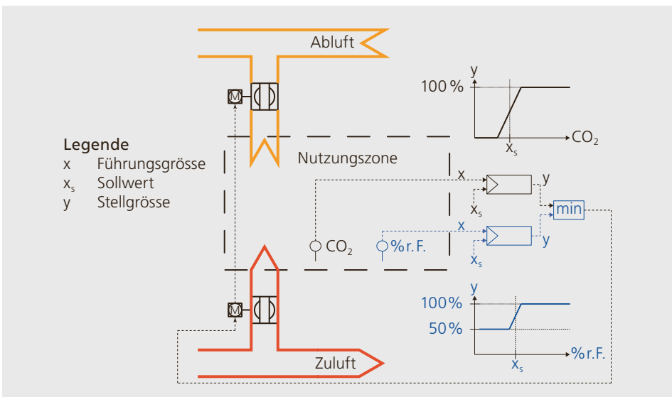
Abbildung 3.23: Beispiel einer Regelstrategie für die Luftmenge während der Heizperiode.
