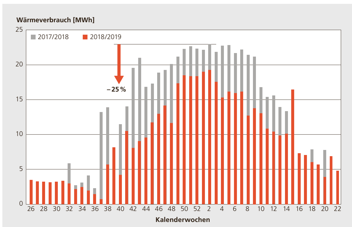
Abbildung 6.8: Entwicklung des fossilen Wärmeverbrauchs im ersten Jahr der Betriebsoptimierung. (Quelle: Böhler, MTU GmbH)
