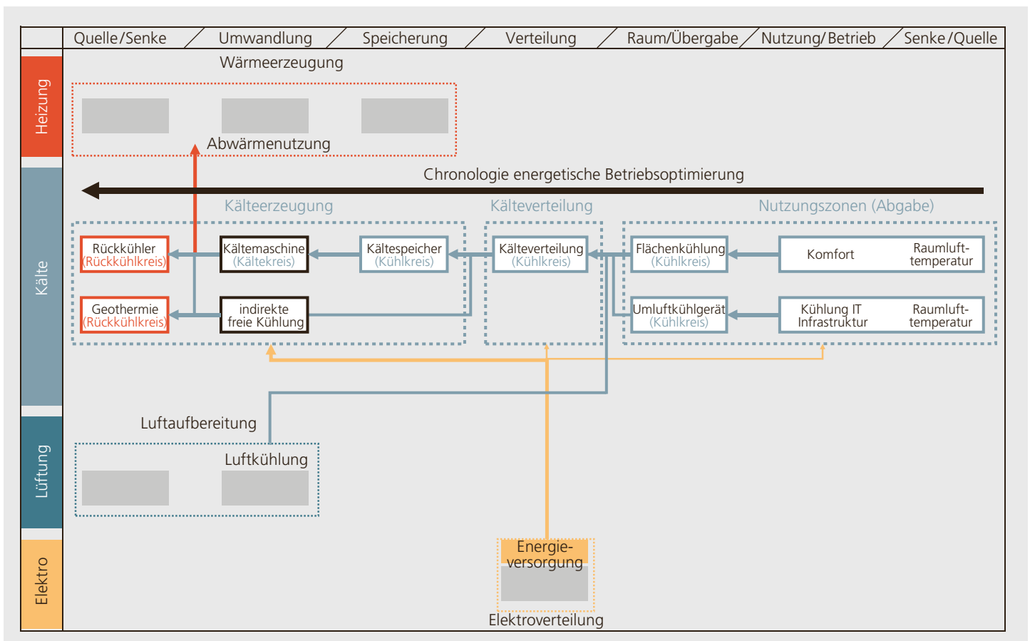
Abbildung 3.37: Beispiel eines typischen Klimakältesystems dargestellt mit Modula GT (SIA 411).
