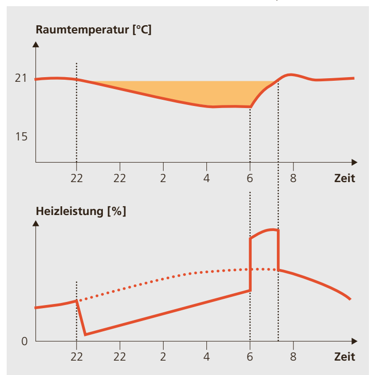
Abbildung 3.7: Massnahme für einen optimierten Absenkebetrieb bei der Wärmeverteilung über Heizkörper.
