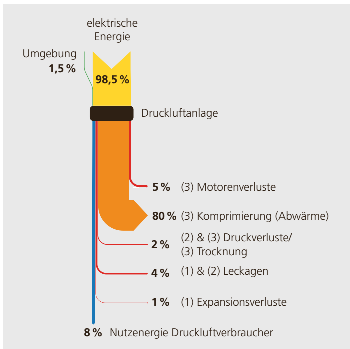
Abbildung 3.43: Energiefluss einer typischen Druckluftanlage vom Verbraucher (1), über die Druckluftverteilung (2) bis zur Druckluftherzeugung (3).
