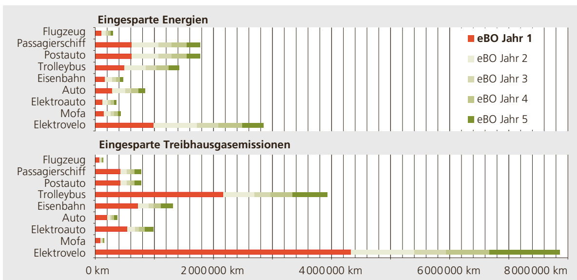
Abbildung 4.7: Vergleich von eingesparter Primärenergie und Treibhausgasemissionen zu gefahrenen Kilometern. Primärenergiefaktoren und Treibhausgasemissionswerte für Heizöl EL sowie den Schweizer Strommix nach KBOB.
