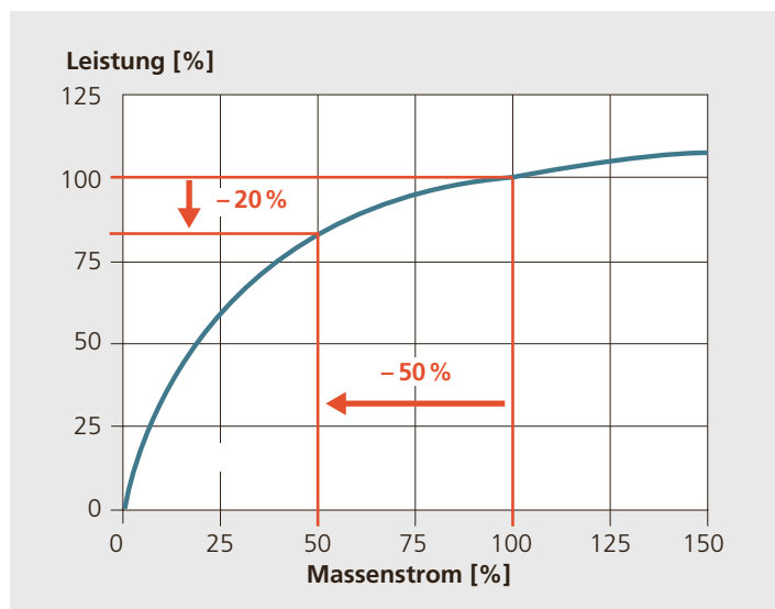
Abbildung 3.9: Wärmeabgabe von Heizkörpern: Wird der Massenstrom reduziert, sinkt die Wärmeabgabe bei Heizkörpern mit hohen Vorlauftemperaturen (> 50°C) unterproportional.
