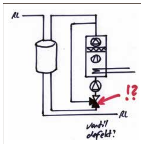
Abbildung 6.7: Prinzipschema Grundwasser-Wärmepumpe mit defektem Regelventil. (Quelle: Böhler, MTU GmbH)
