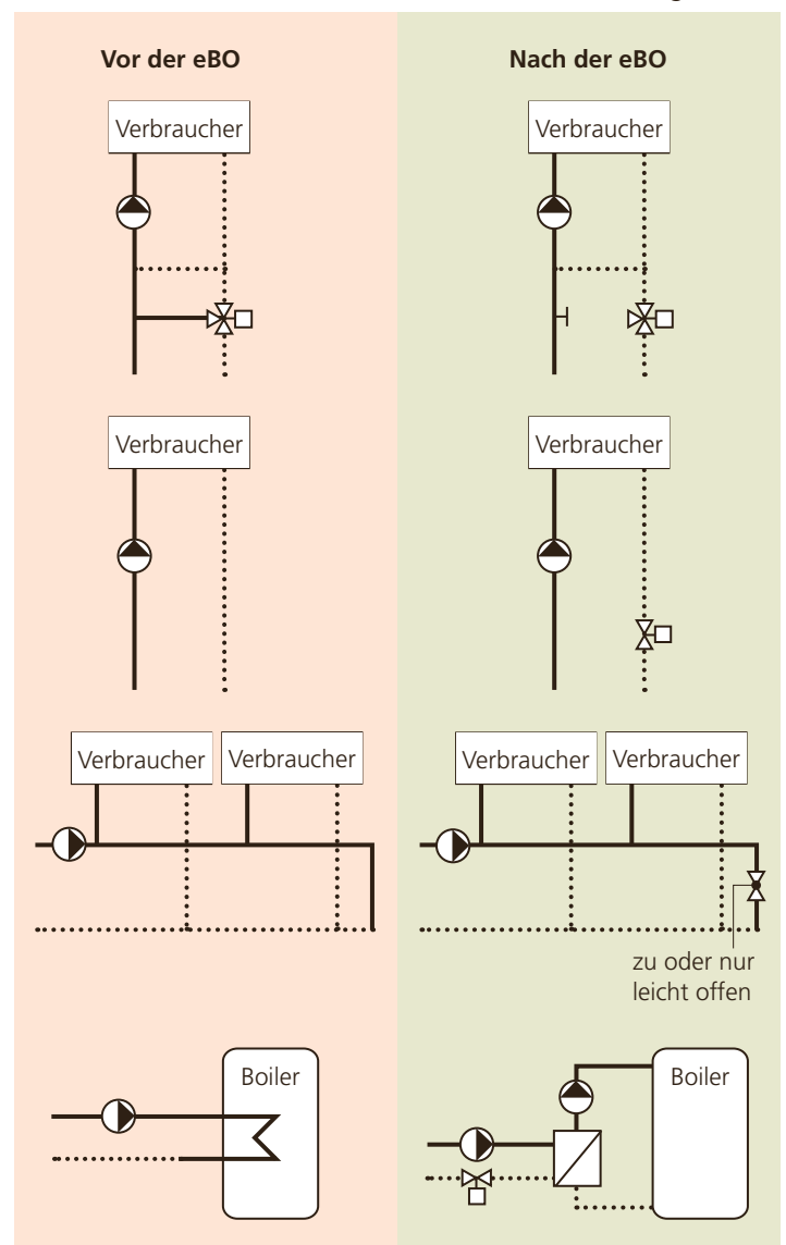
Abbildung 3.54: Drosselschaltungen ermöglichen tiefe Rücklauftemperaturen. (Quelle: Angelo Lozza, Lozza Energie)
