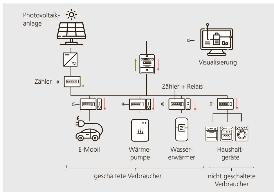
Abbildung 3.57: Lastmanagement-systeme steuern verbraucherabhängig vom produzierten Strom und steigern so den Eigenverbrauch. (Quelle: David Zogg, FHNW)
