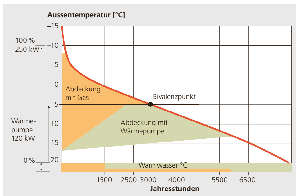
Abbildung 3.13: Beispiel für den Bivalenzpunkt im Summenhäufigkeitsdiagramm.
