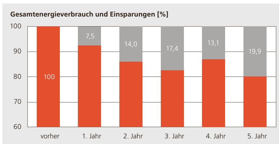
Abbildung 6.10: Technische Berufsschule, Zürich – Einspareffekte beim Energieverbrauch durch Betriebsoptimierung. (Quelle: Energo)
