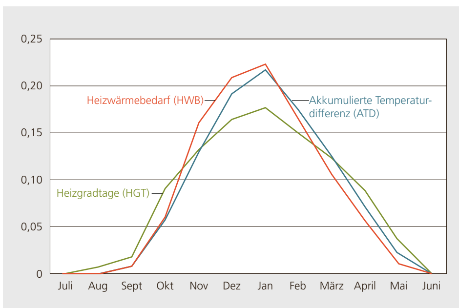
Abbildung 4.28: Vergleich Heizgradtage (HGT) und akkumulierte Temperaturdifferenz (ATD) zum effektiven Heizwärmebedarf (HWB). (Quelle: Gerhard Zweifel, SIA)
