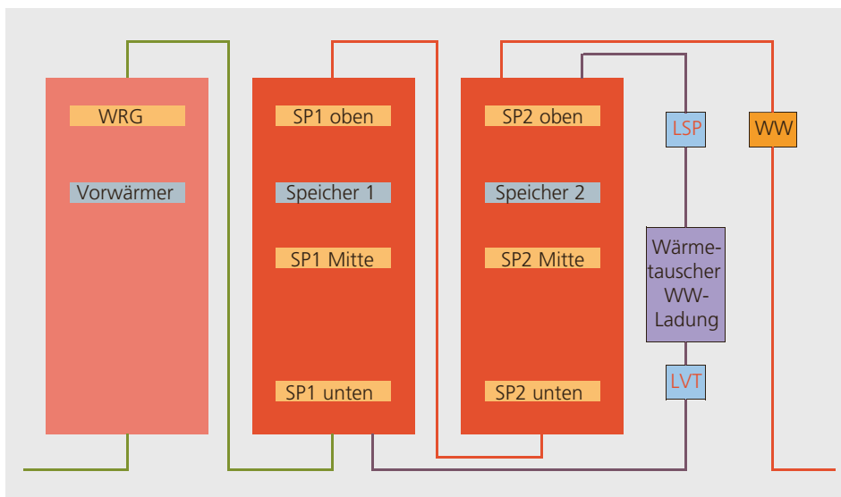
Abbildung 3.17: Schema für Messungen an einer Warmwasserversorgung. (Quelle: S. Murchini, Büro für Messtechnik)
