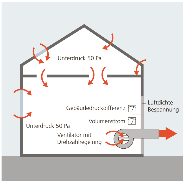
Abbildung 2.9: Schema Blower- Door-Messung.
