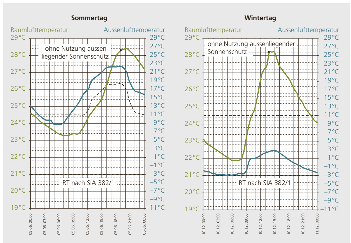
Abbildung 3.33: Raumtemperaturen Sommer und Winter in einem Büro ohne Nutzung des ausenliegenden Sonnenschutzes.
