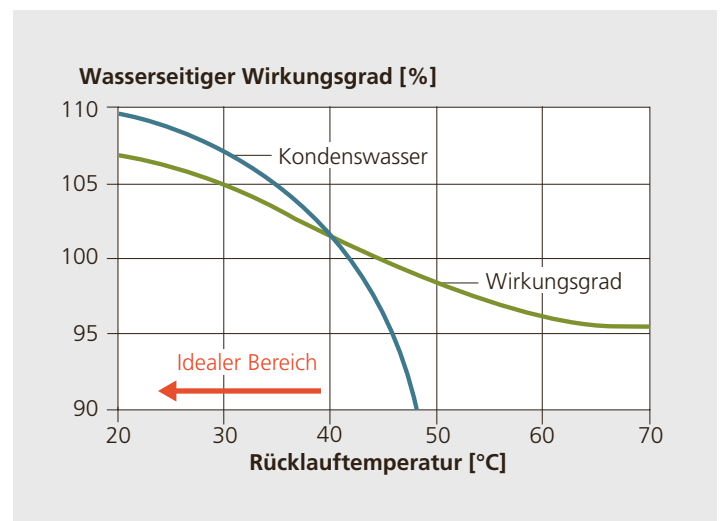
Abbildung 3.11: Heizkesselwirkungsgrad bei Gasbrennwertkesseln in Abhängigkeit der Rücklauftemperatur.
