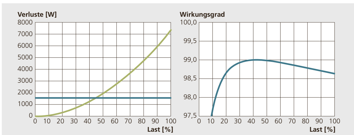
Abbildung 3.56: Verluste eines 630-kVA-Trockentransformators. (Quelle: Siemens)
