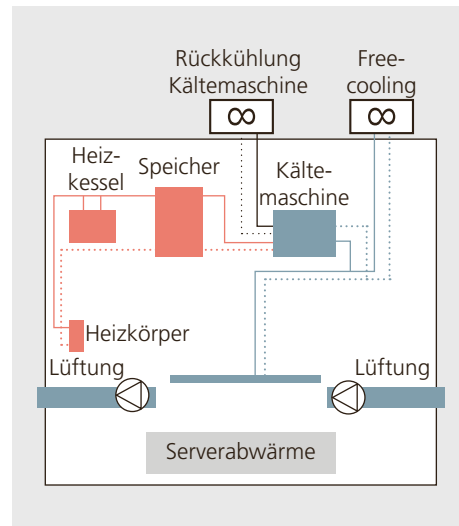
Abbildung 3.53: Beispiel einer Anlage mit Serverraumkühlung. (Quelle: Angelo Lozza, Lozza Energie und Gebäudetechnik)
