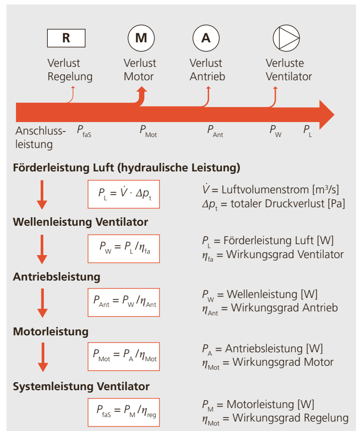
Abbildung 3.27: Leistungsdiagramm zur Ermittlung des SFP eines Ventilators.
