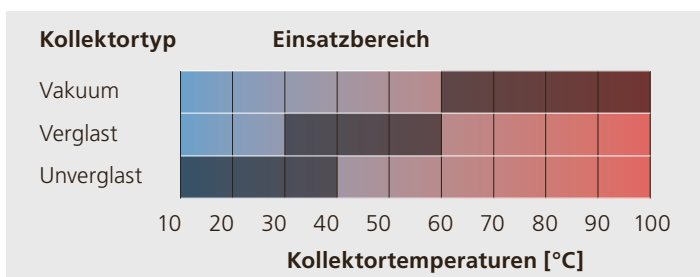
Abbildung 3.59: Einsatzbereich Kollektortypen bezogen auf das Temperaturniveau. (Quelle: energie-soaire.ch)
