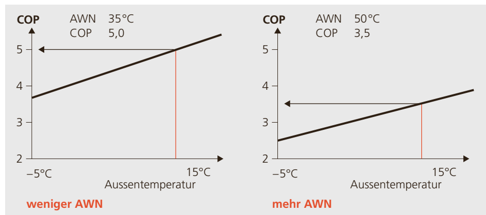
Abbildung 3.52: AWN aus Kälteanlagen mit verschiedenen Temperaturniveaus.
