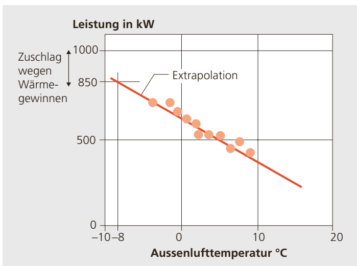
Abbildung 3.10: Ermittlung der notwendigen Auslegungswärmeleistung im Gebäudebestand mittels Extrapolation von gemessenen Wärmeleistungen.
