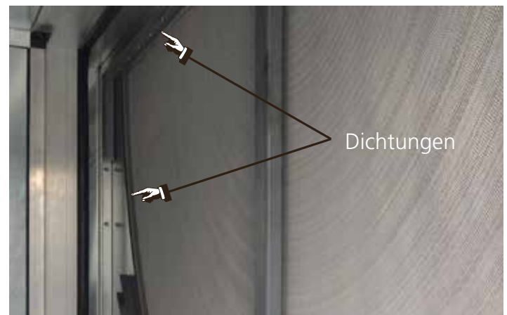
Abbildung 3.30: Bürstendichtungen WRG-Rotationssystem.
