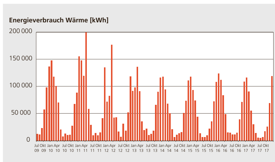
Abbildung 6.14: Energieverbrauch Wärme, Sporthalle Wankdorf, witterungs- bereinigt: 2013 wurden die Lüftungsanlagen angepasst, 2013/2014 wurden die automatischen Türschliesser instal- liert. (Quelle: Ergo)
