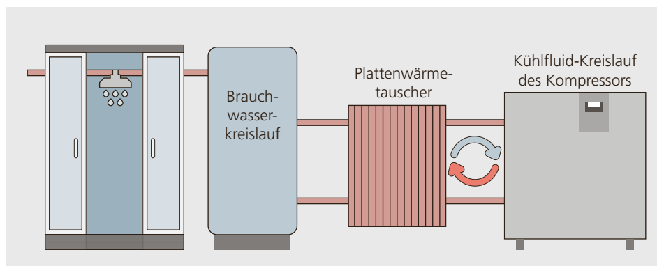
Abbildung 3.20: Schematisch Einbindung der WRG einer Druckluftanlage in die Warmwasserversorgung.
