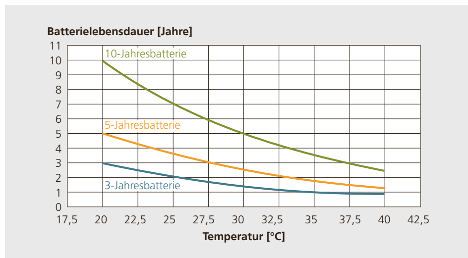
Abbildung 3.46: Lebensdauer von USV-Batterien ver- sus Umgebungstem- peratur. (Quelle: Control Enginee- ring)
