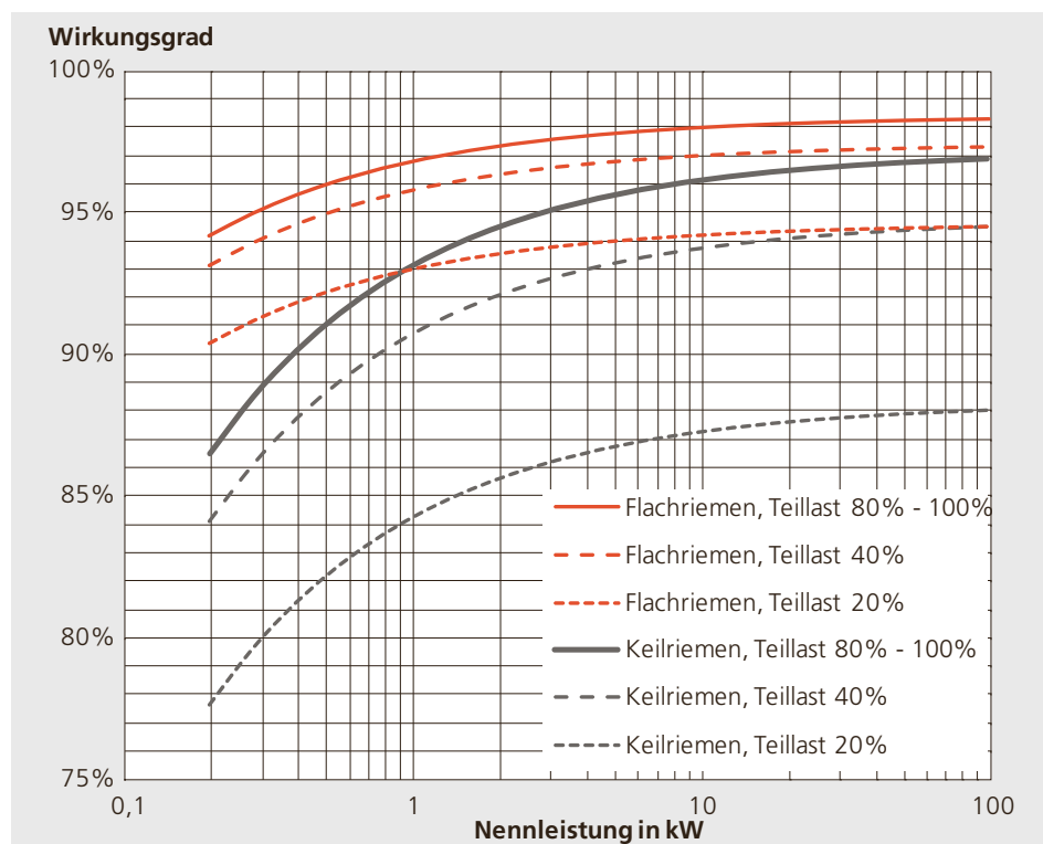
Abbildung 3.28: Transmissionswirkungsgrade von Keil- und Flachriemen je nach Nennleistung des Motors und Lastanteil (Antriebe mit 1 Riemen), (Quelle: EnergieSchweiz, topmotors.ch; Merkblatt 24, November 2012)
