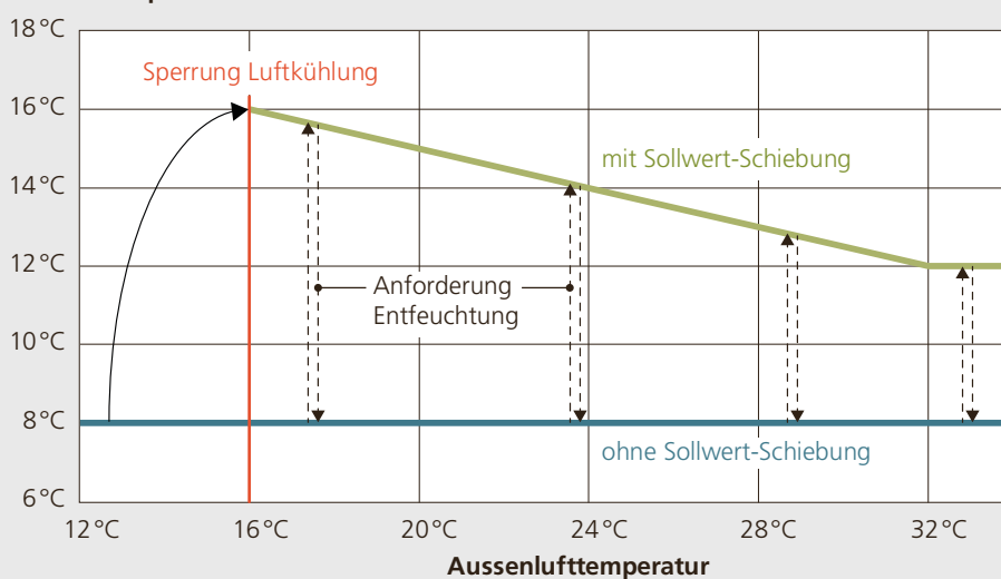
Vorlauftemperatur Kühlwasser
