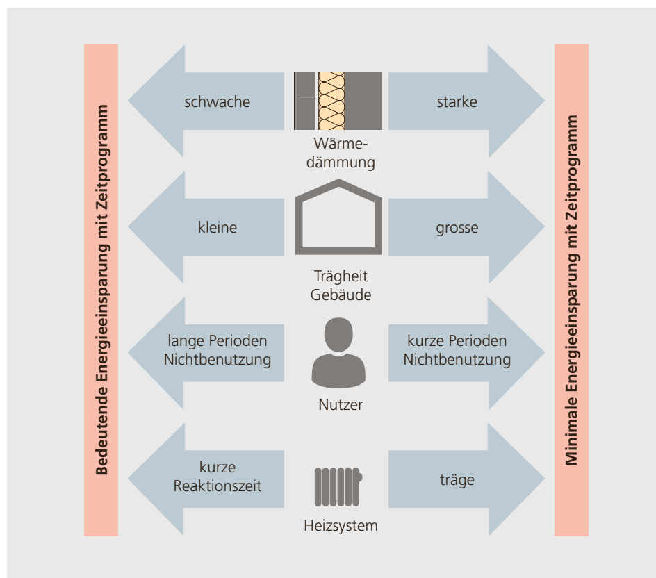
Abbildung 3.8: Wie viel Energie sich durch Nachtabsenkung sparen lässt, hängt von verschiedenen Faktoren ab.
