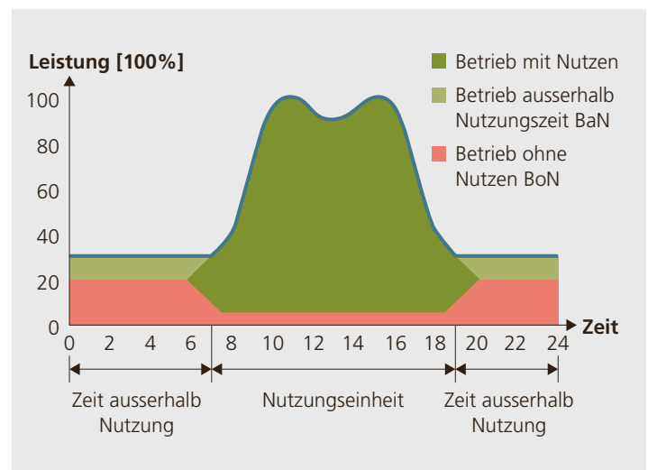
Abbildung 3.48: Elektroinstallationen: BaN (Betrieb ausserhalb der Nutzungszeit) und BoN (Betrieb ohne Nutzen). (Quelle: Swiss Energy Codes – Revision SIA 380/4, Teilprojekt 7: Verlastungsoptimierte Elektroinstallationen)
