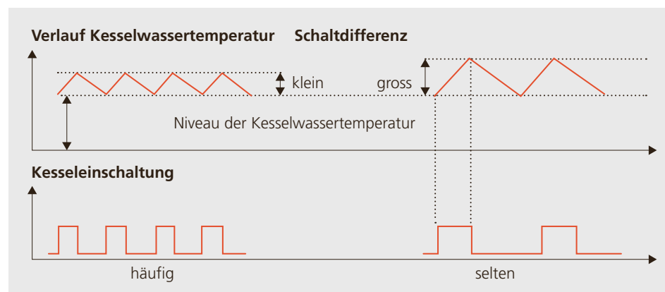
Abbildung 3.12: Auswirkung einer zu kleinen Schaltdifferenz (links): Der Brenner schaltet damit häufig ein und aus, die Verluste steigen.
