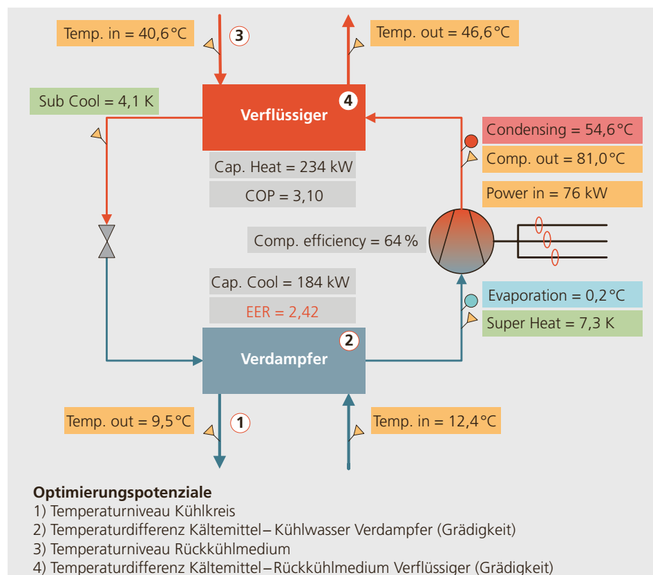
Abbildung 3.41: Mit KlimaCheck gemessene Temperaturen und daraus ermittelte Leistungen im Vollastbetrieb.
