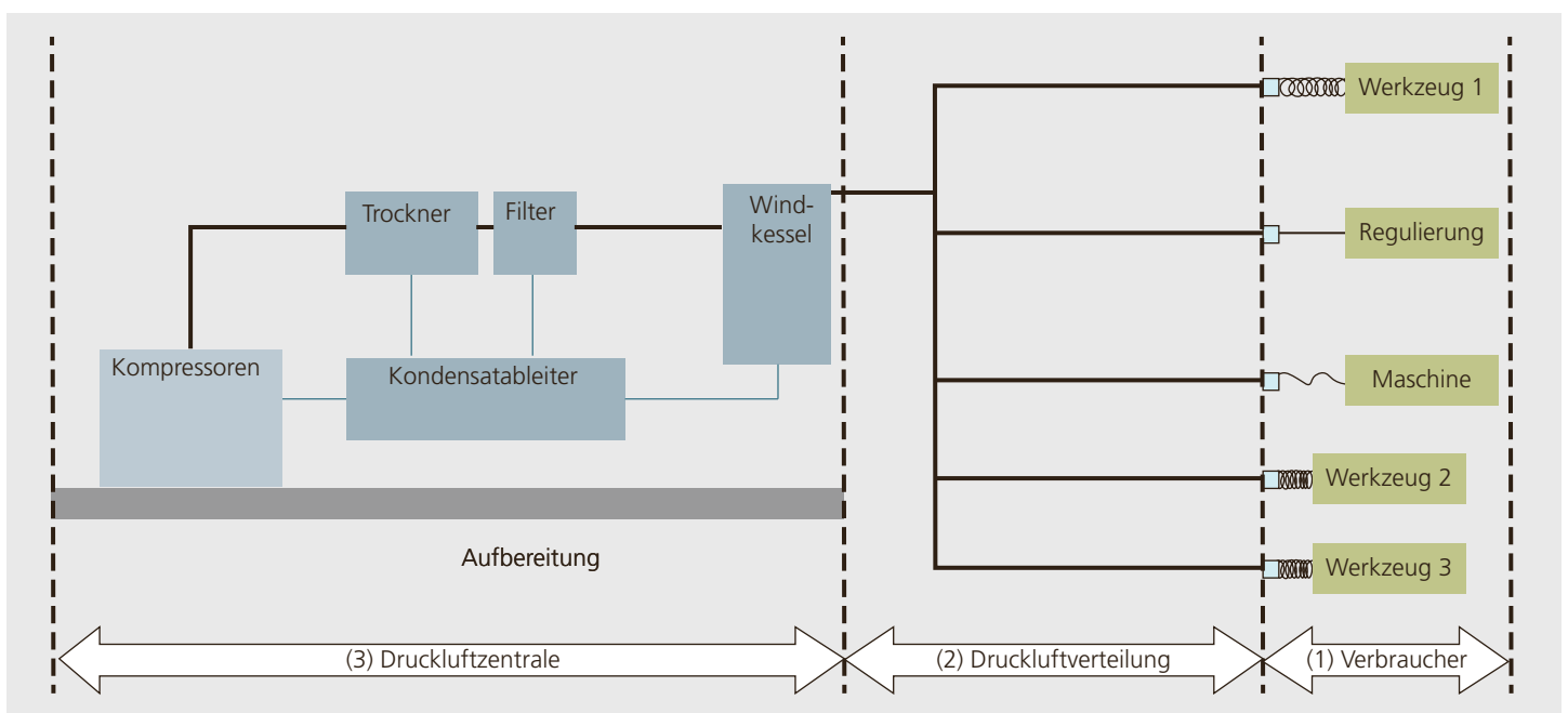
Abbildung 3.44: Schema einer Druckluftanlage mit Verbraucher (1), Druckluftverteilung (2) und Druckluftherzeugung (3).
