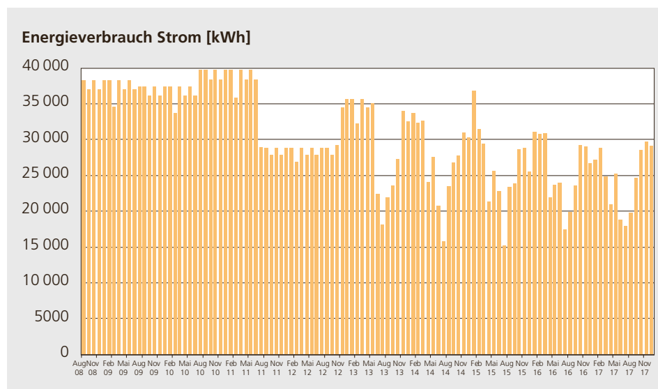
Abbildung 6.13: Energieverbrauch Strom, Sporthalle Wankdorf: 2011 Teilersatz der Hallenbeleuchtung, 2013 Anpassung der Lüftungsanlage. (Quelle: Ergo)
