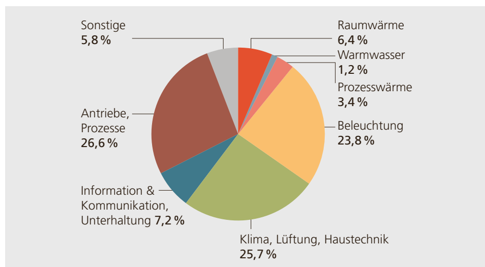
Abbildung 3.1: Elektrizitätsverbrauch nach Verwendungszweck im Schweizer Dienstleistungssektor 2017. (Quelle: BFE 2018)
